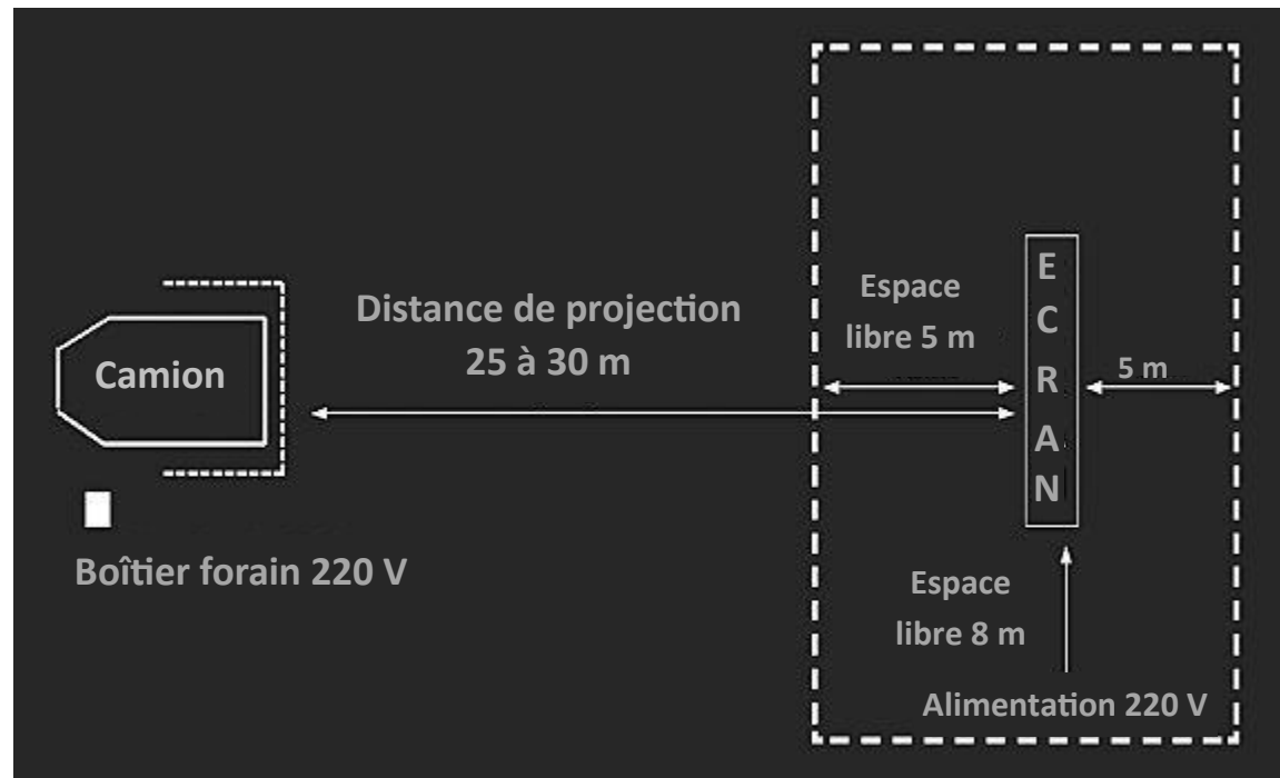
Plan : Ecran Gonflable de 10mx8m
